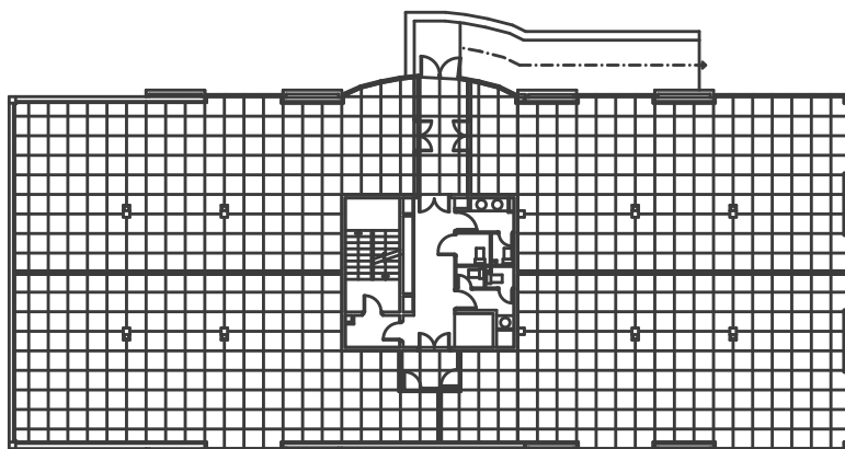
PLANTA SEMISOTANO
