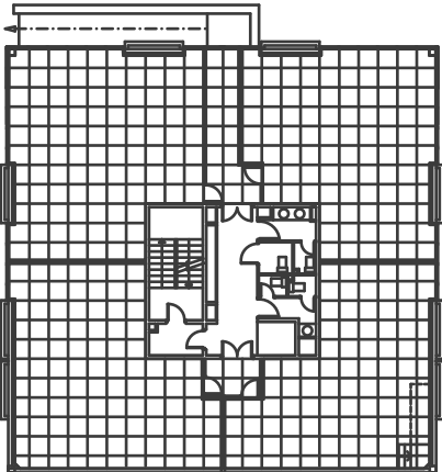
PLANTA SEMISOTANO
