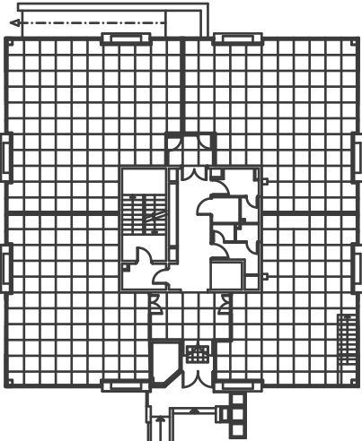
PLANTA BAJA
